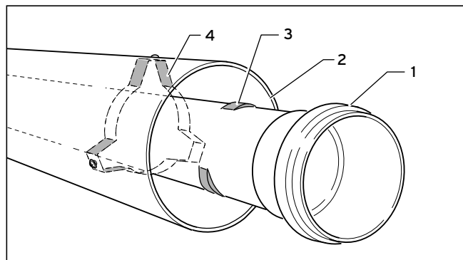
Obr. 4.55 Uvoľnenie potrubia odvodu spalín
