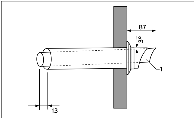
Obr. 4.27 Montáž vodorovnej priechodky stenou
