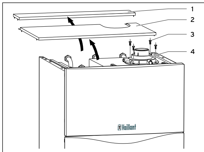
Obr. 5.1 Montáž prípojky zariadenia
