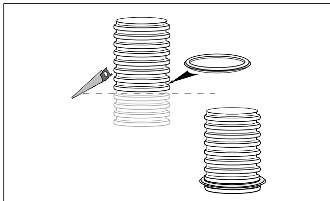
Obr. 4.45 Skrátenie flexibilného odvodu spalín a montáž tesnenia
