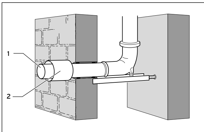
Obr. 4.39 Prevádzka závislá na vzduchu v miestnosti
