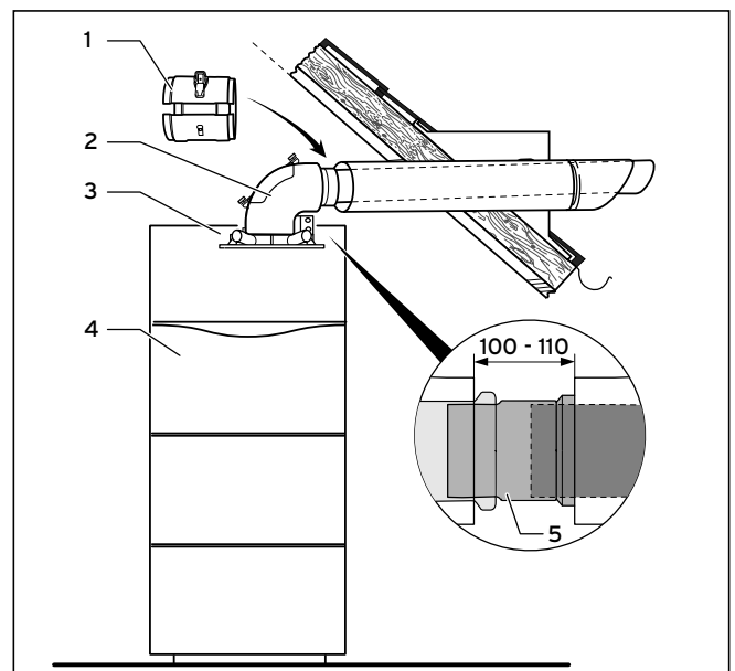
Obr. 4.29 Priama inštalácia
