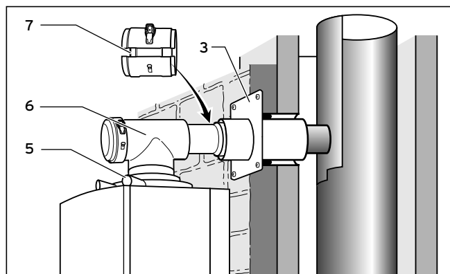
Obr. 5.14 Montáž zariadenia
