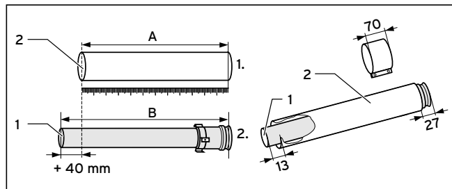
Obr. 4.56 Skrátenie rúr
