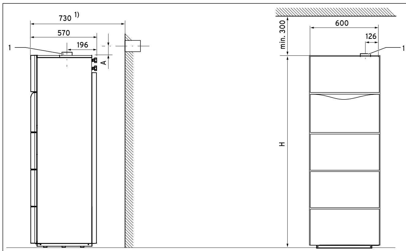
Obr. 3.1 Montážne rozmery (v mm)
