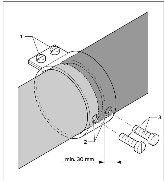
Obr. 5.39 Montáž vzduchových príchytiek
