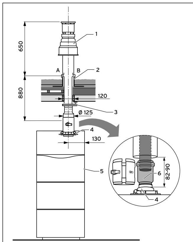
Obr. 5.5 Montáž zariadenia a prechodu plochou strechou
