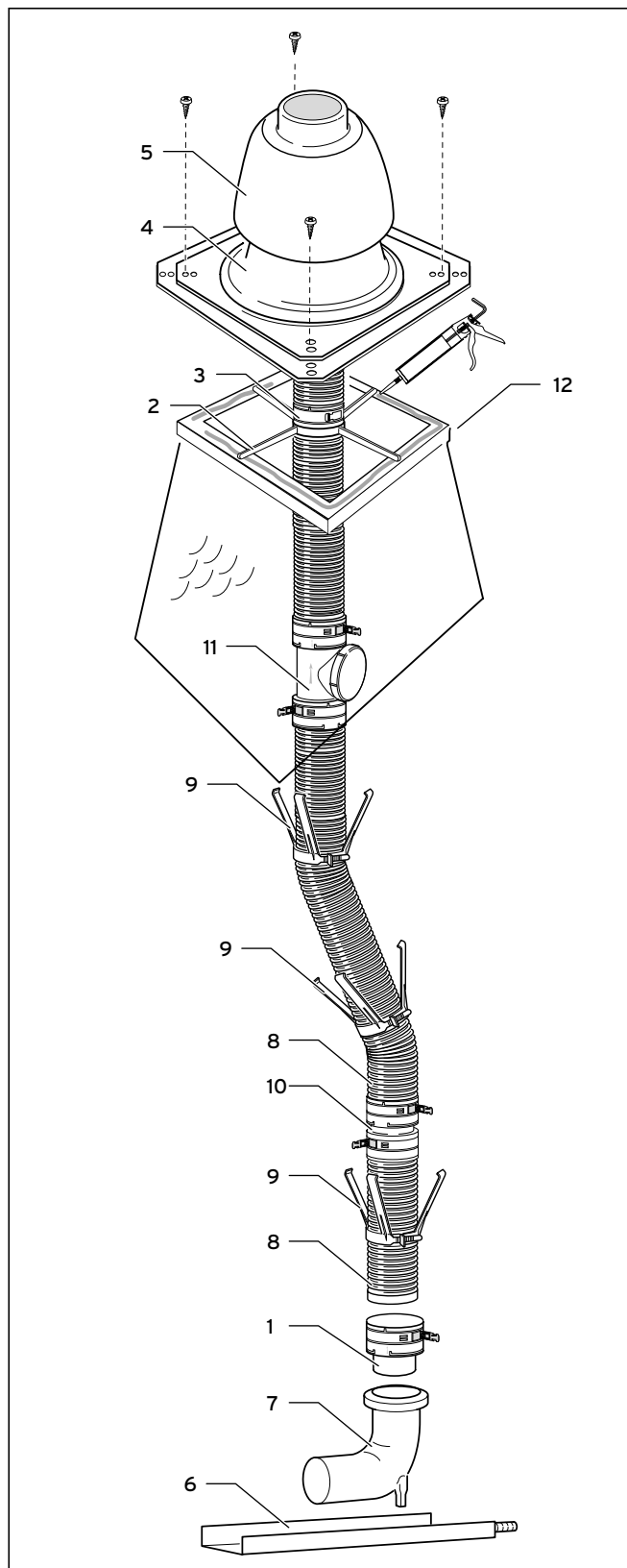
Obr. 5.28 Systémová skladba flexibilního odvodu spalín
