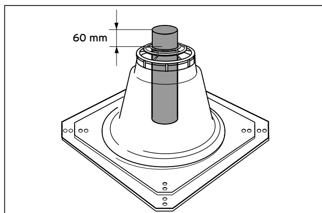
Obr. 4.36 Dĺžka vrchnej trubky odvodu spalín
