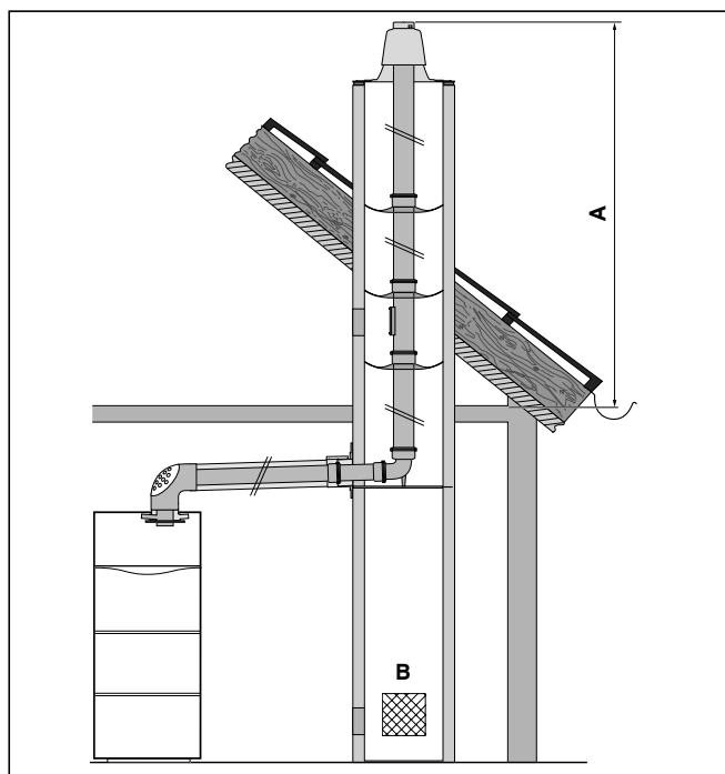
Obr. 4.33 Príklad montáže závislej od vzduchu miestnosti
