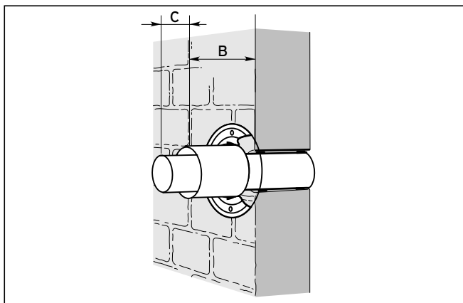
Obr. 3.2 Prevádzka závislá na vzduchu v miestnosti
