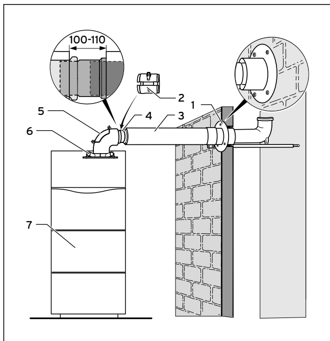
Obr. 4.41 Montáž vodorovného odseku
