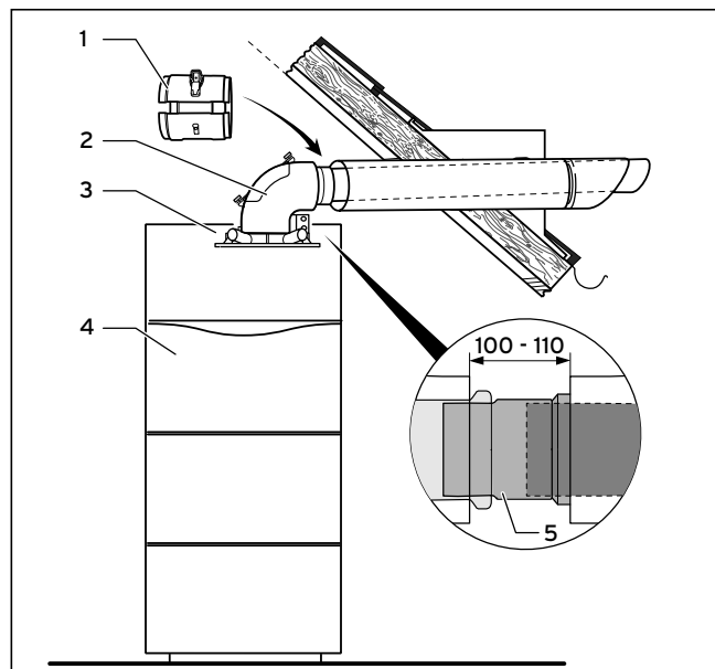
Obr. 4.12 Priama inštalácia
