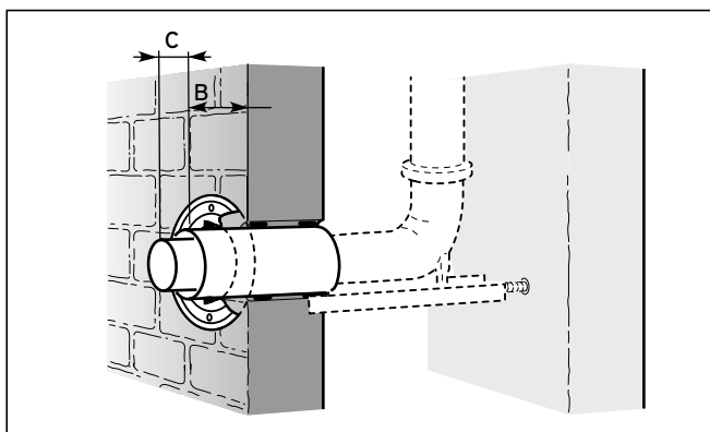
Obr. 3.3 Prevádzka nezávislá na vzduchu v miestnosti
