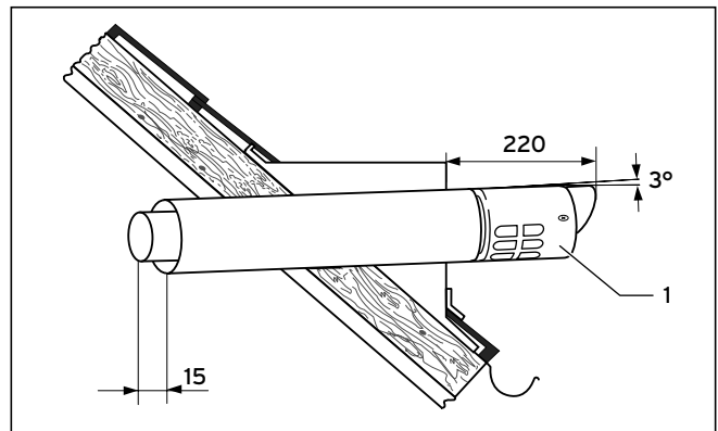
Obr. 5.7 Montáž strešnej prechodky
