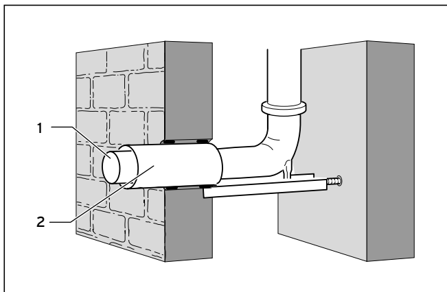
Obr. 4.40 Prevádzka nezávislá na vzduchu v miestnosti
