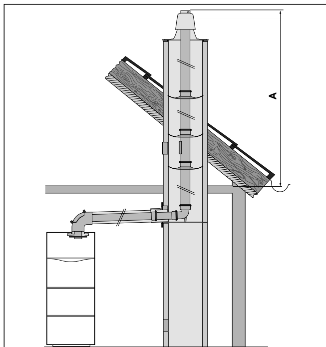
Obr. 4.32 Príklad montáže nezávislej od vzduchu miestnosti
