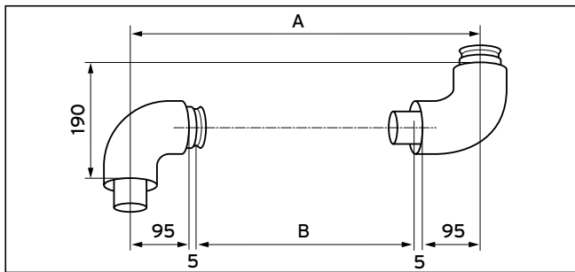
Obr. 5.42 Montáž 87° oblúkov
