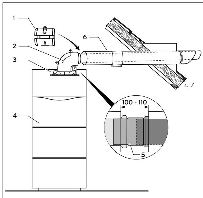
Obr. 4.21 Vzdialená inštalácia
