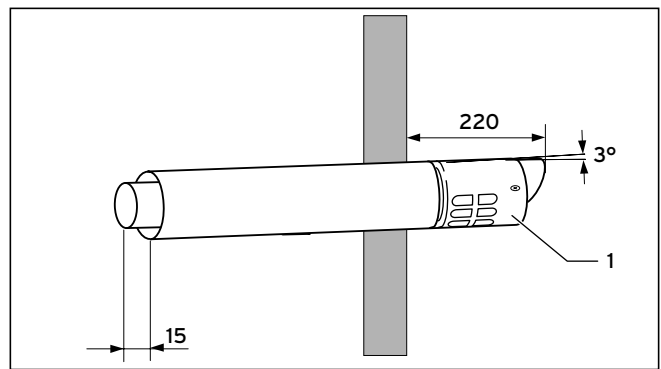
Obr. 5.8 Vodorovná stenová prechodka
