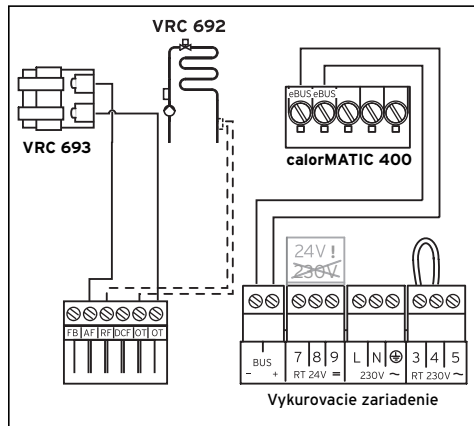
Obr. 10.1 Elektrické pripojenie
