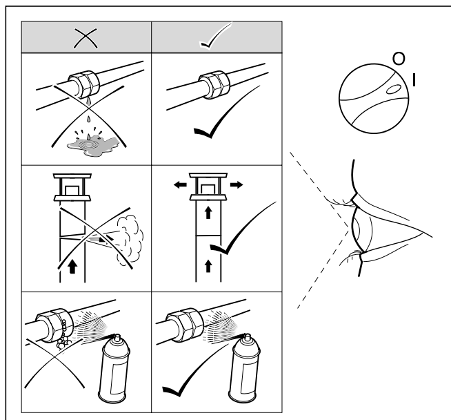
Obr. 8.3 Kontrola funkce
