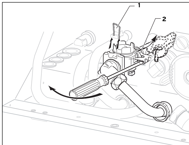
Obr. 4.9 Sejmутí pružné spony a svorky
