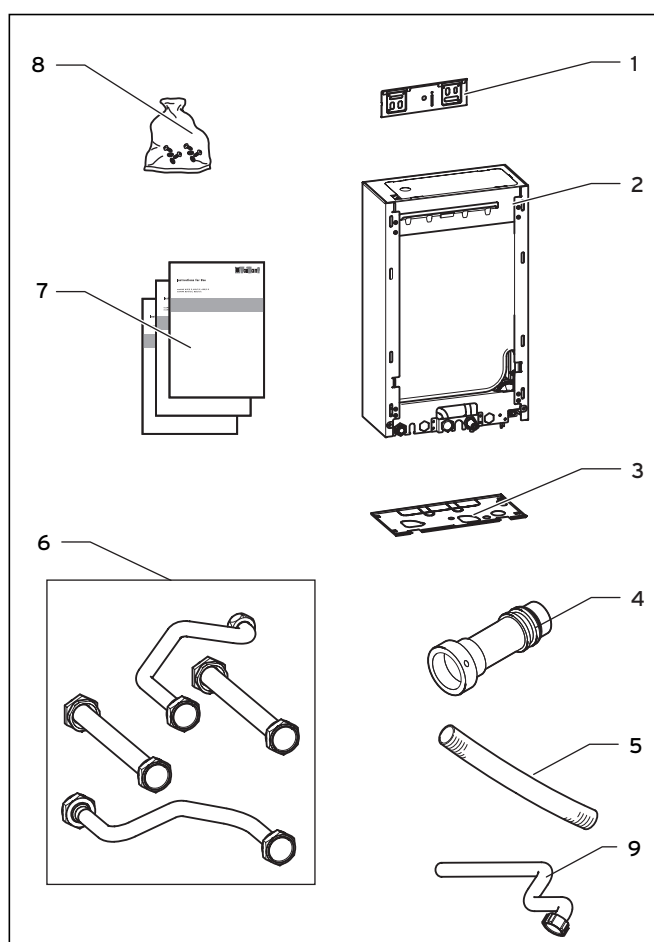
Obr. 4.1 Rozsah dodávky
