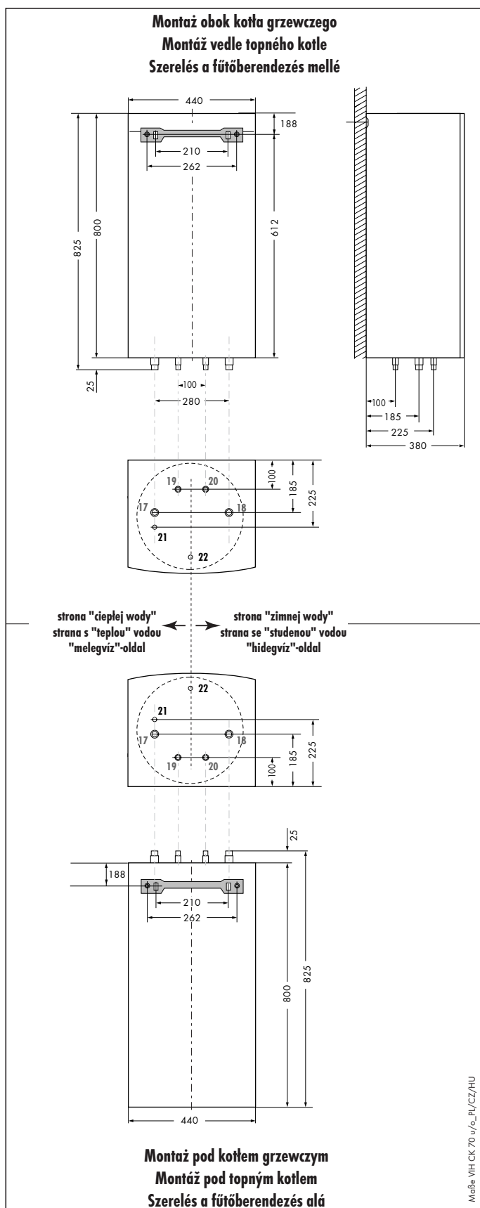
Rys. 5.2 Wymiary podgrzewacza zasobnikowego VIH CK 70.
