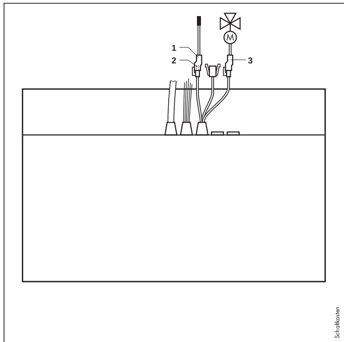
Rys. 5.3 Połączenie elektryczne. Obr. 5.3 Propojeni 5.3 ábra: Elektromos bekötés
