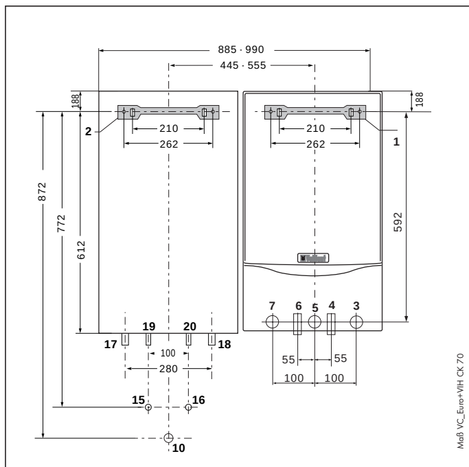
Rys. 4.2 Montaż obok konwencjonalnych kotłów grzewczych.
