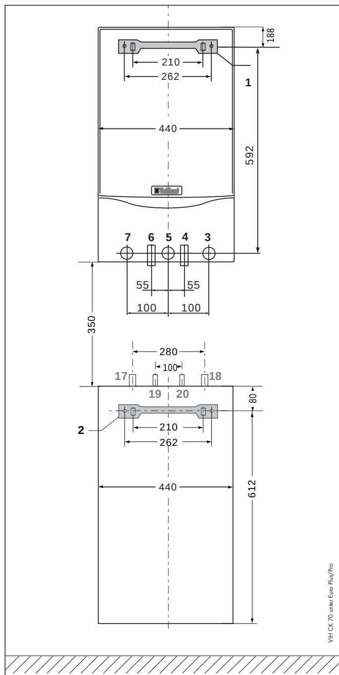
Rys. 4.4. Montaż pod konwencjonalnymi kotłami grzewczymi.
