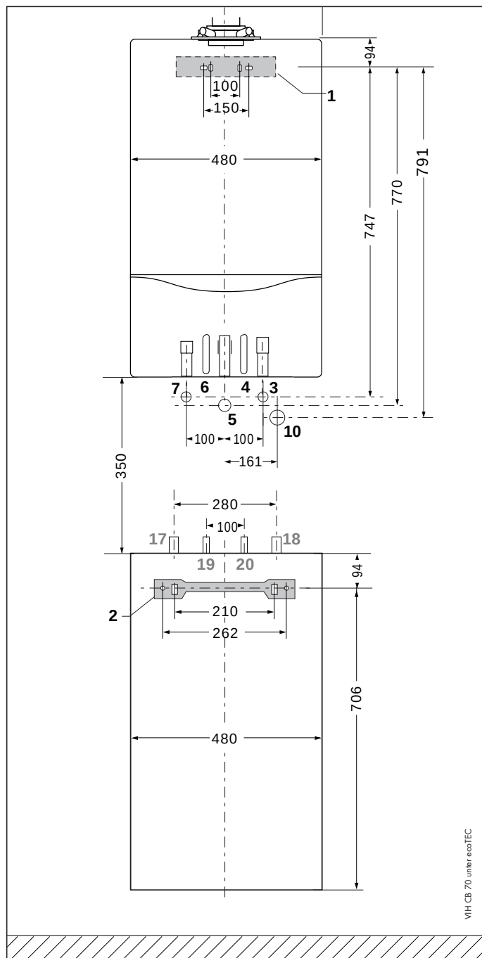
Rys. 4.3. Montaż pod kondensacyjnymi kotłami grzewczymi.
