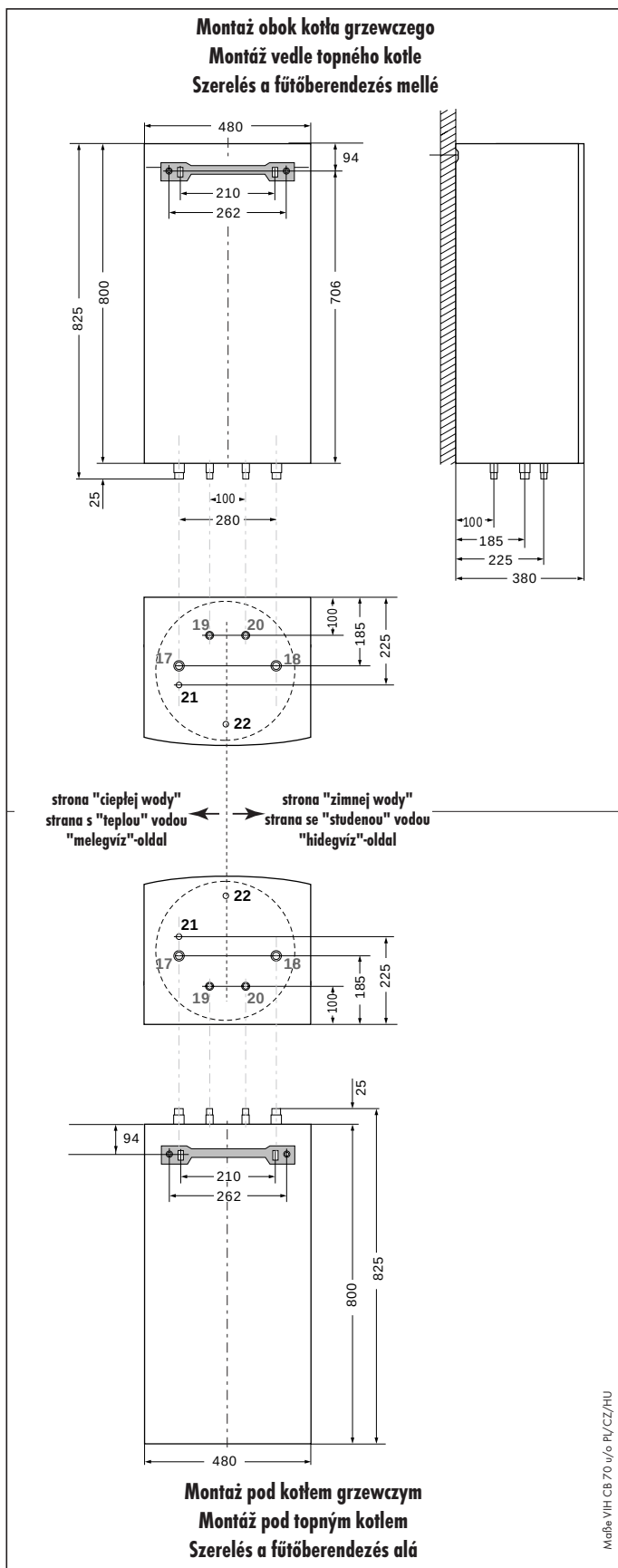
Rys. 5.1 Wymiary podgrzewacza zasobnikowego VIH CB 70.
