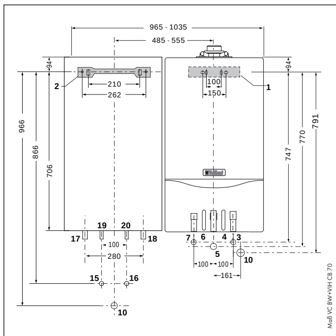
Rys. 4.1 Montaż obok kondensacyjnych kotłów grzewczych.
