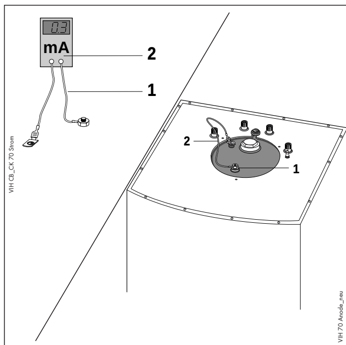
Rys. 6.1 Konserwacja anody ochronnej Obr. 6.1 Údržba ochranné anody 6.1 ábra: A védőanód karbantartása
