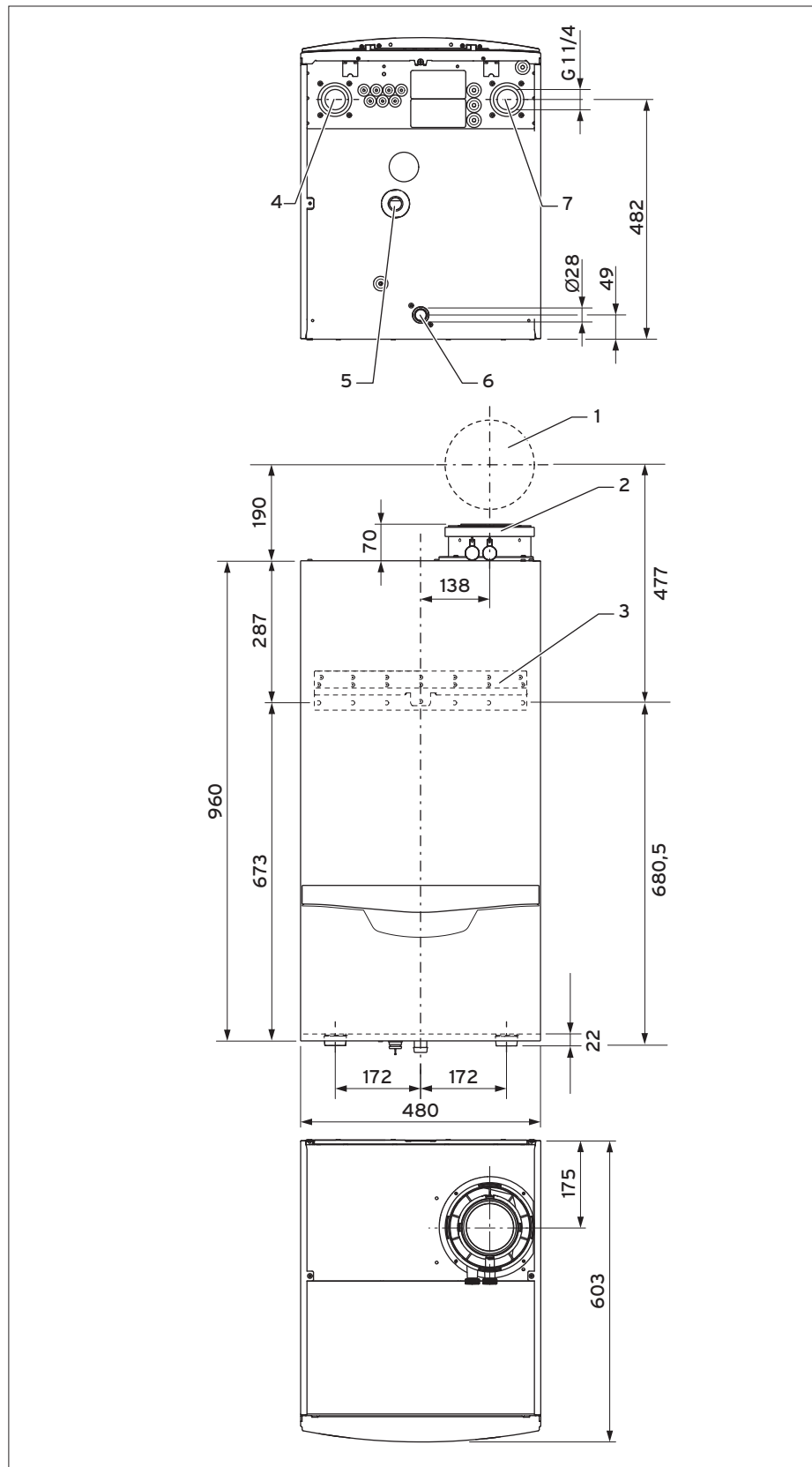
Schéma s rozměry a připojovací míry
