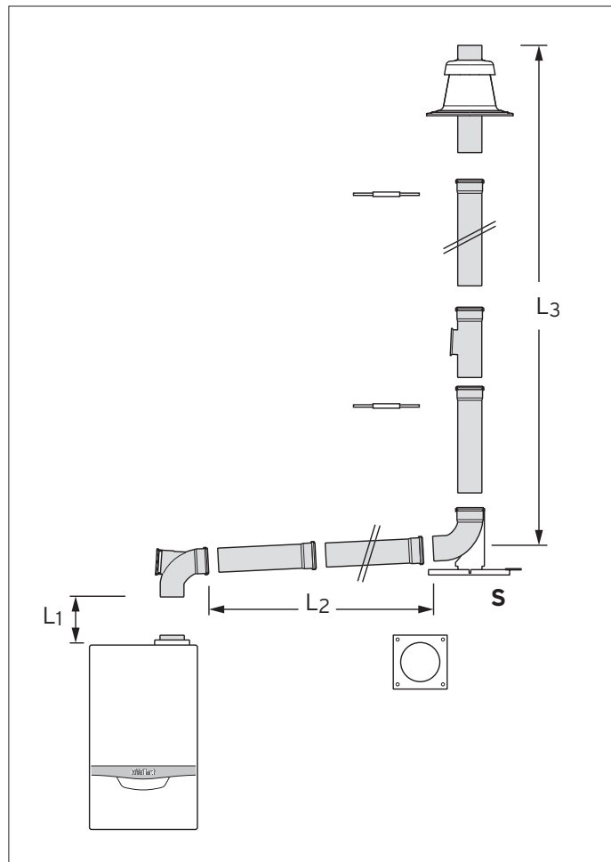
Přípojka na odvod spalín DN 110 PP (pevný) v šachtě (příklad použití)
