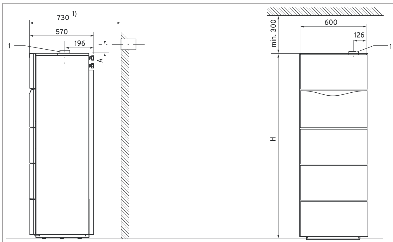
Montážne rozmery (v mm)
