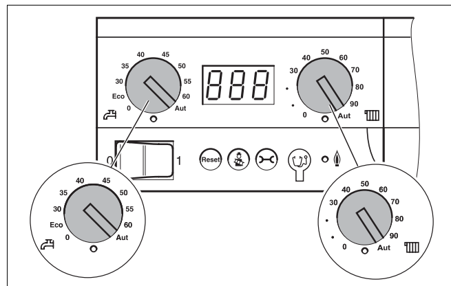
Obr. 3 Nastavenie regulátora
